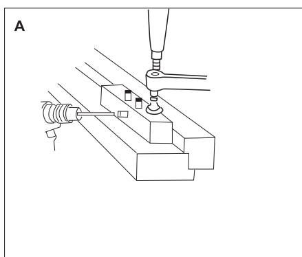
企口門用打孔模具
