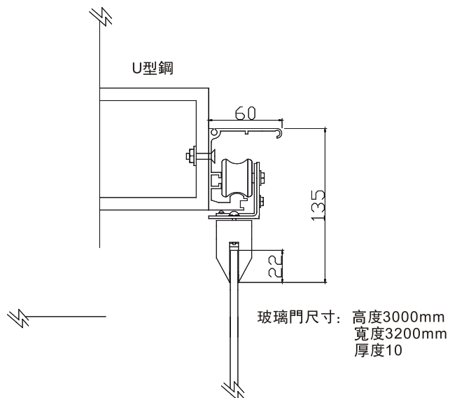
雙輪滑輪組
