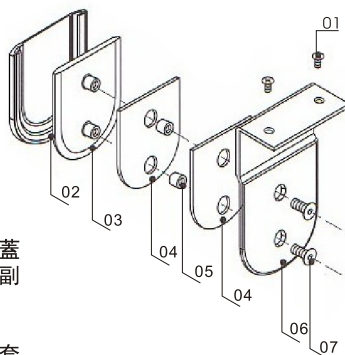
玻璃固定副安裝示意圖
