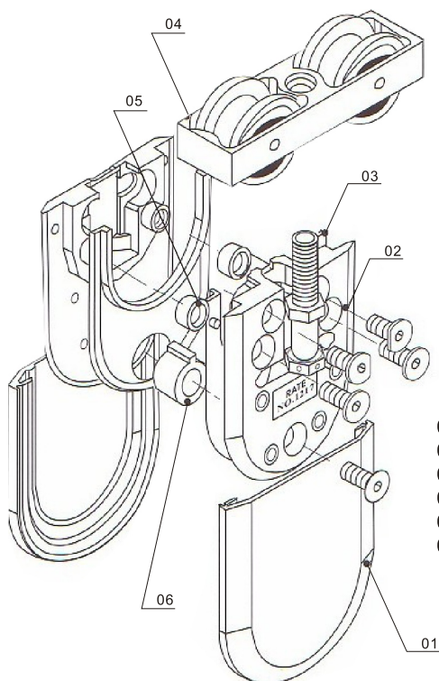
玻璃移動副安裝示意圖
