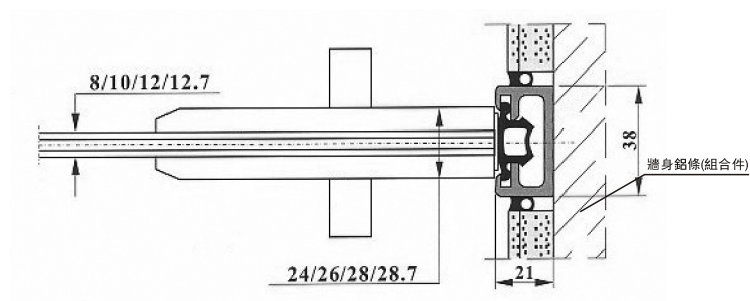
單玻璃移门锁安裝尺寸圖
