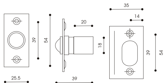
Solid brass ball catch/碰珠(實心銅)
