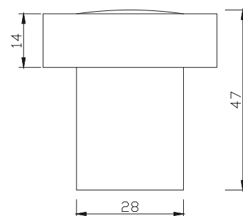
Brass door stopper/門碰(銅)
