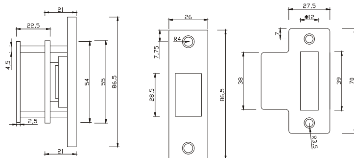
Solid brass ball catch/碰珠(實心銅)
