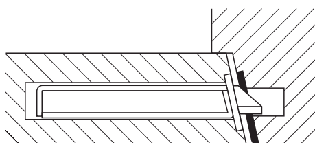
平口斜邊門鎖體安裝示意圖 (護片居中，傾斜固定于鎖體盒上)
