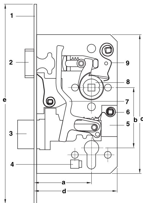
鎖體零部件名稱 及主要尺寸
