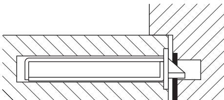
平口門鎖體安裝示意圖 (護片居中固定于鎖體盒上)
