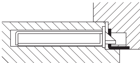
企口門鎖體安裝示意圖 (護片偏心固定于鎖體盒上)
